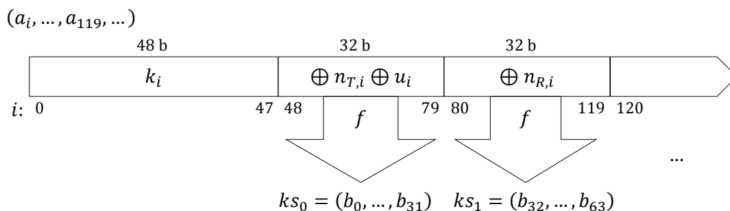
Obrázek 4.4-2 Vývoj vnitřního stavu šifry
