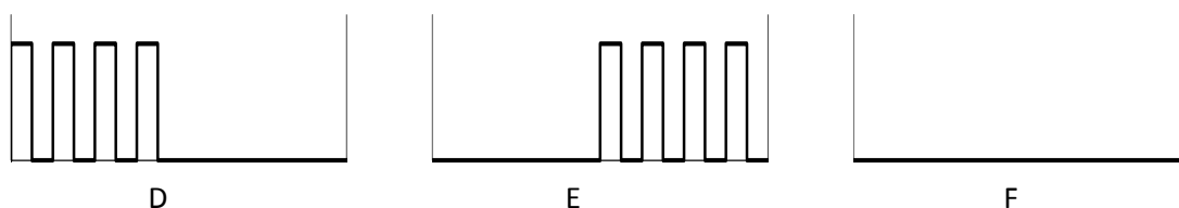
Obrázek 2.5-3 Kódování bitů z transpondéru do terminálu
