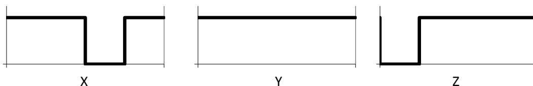
Obrázek 2.5-1 Kódování bitů z terminálu do transpondéru
