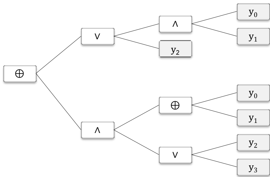
Obrázek 5.4-2 Strom funkce f_b
