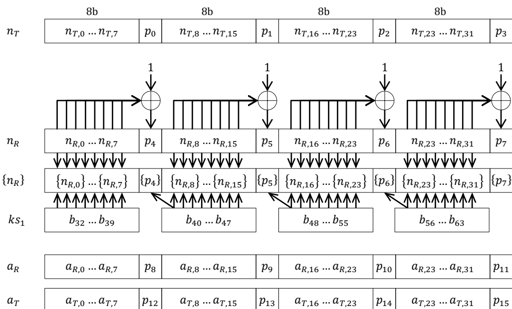
Obrázek 5.1-1 Výpočet a šifrování paritních bitů
