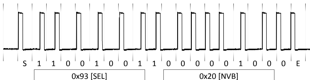
Obrázek 2.5-2 Záznam výběru transpondéru terminálem
