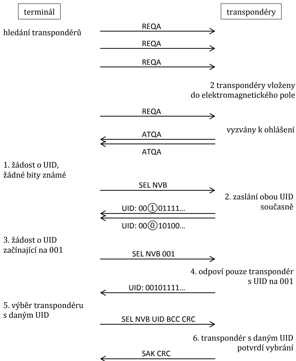
Obrázek 2.6-1 Antikolizní protokol
