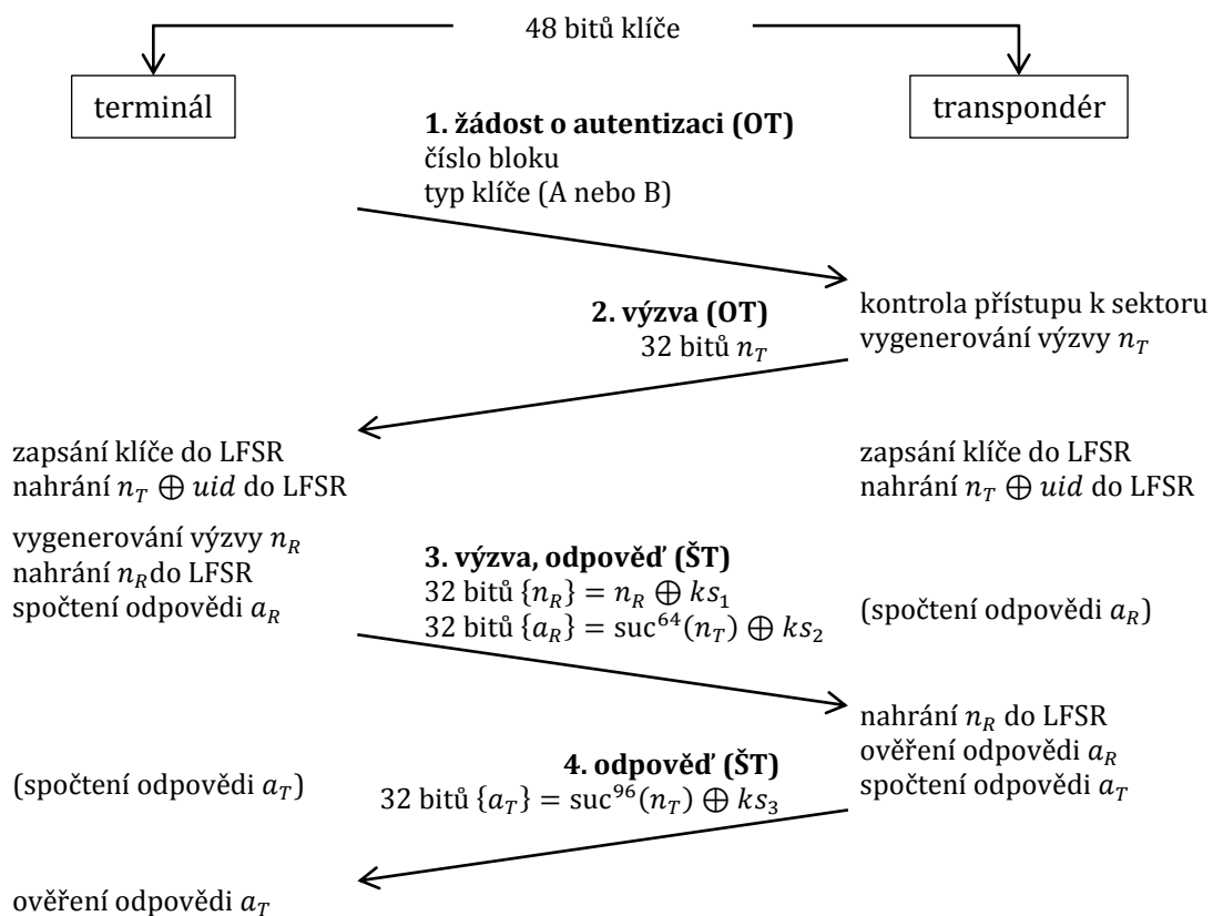
Obrázek 4.4-1 Schéma autentizačního protokolu
