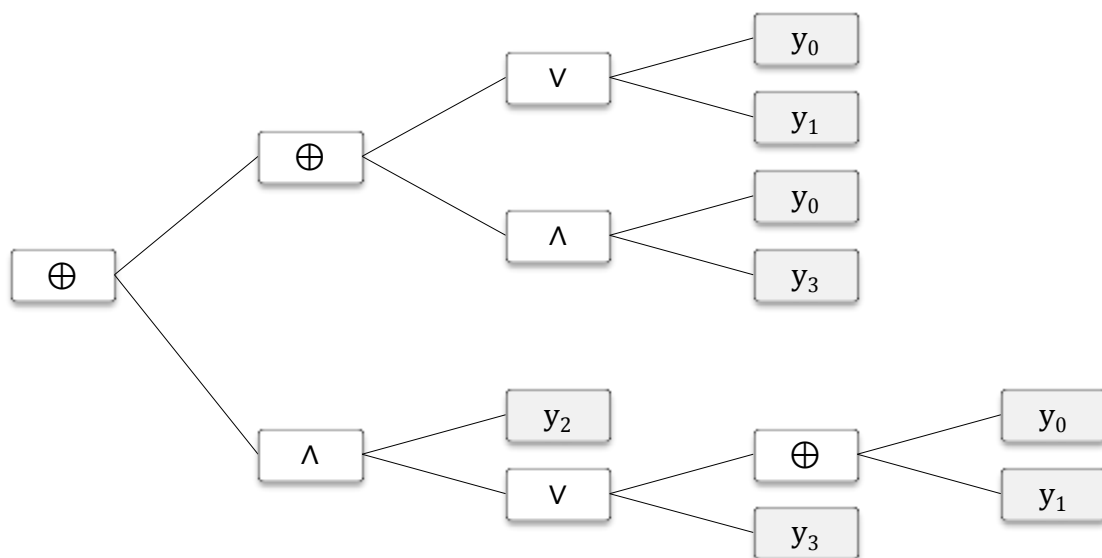
Obrázek 5.4-1 Strom funkce f_a
