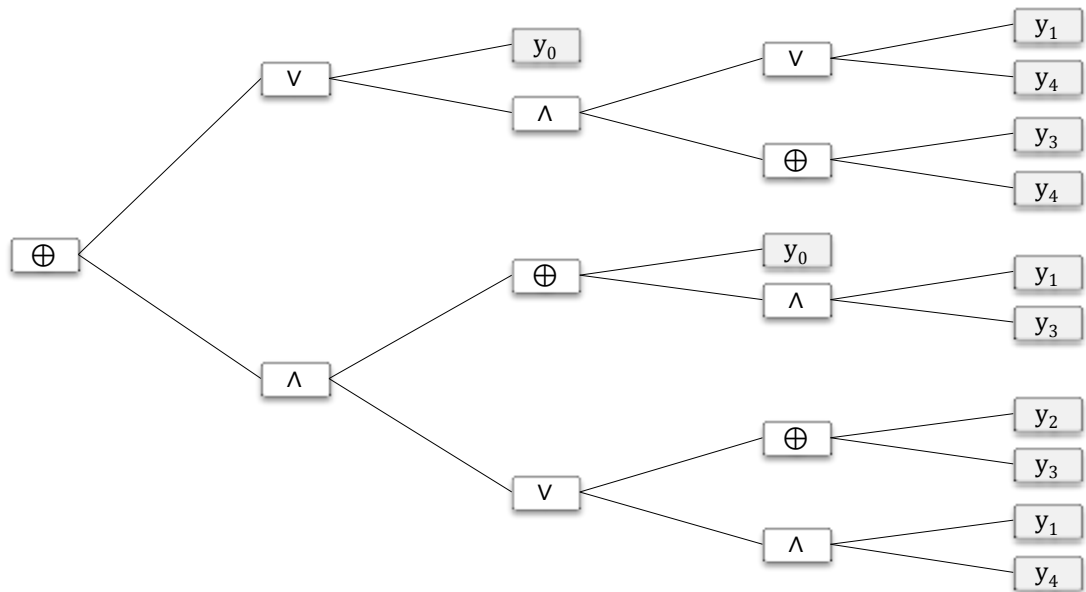
Obrázek 5.4-3 Strom funkce f_c
