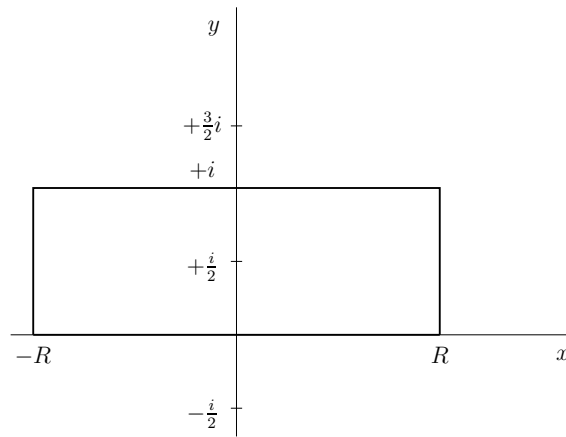
Obrázek 1: Křivka \gamma .
