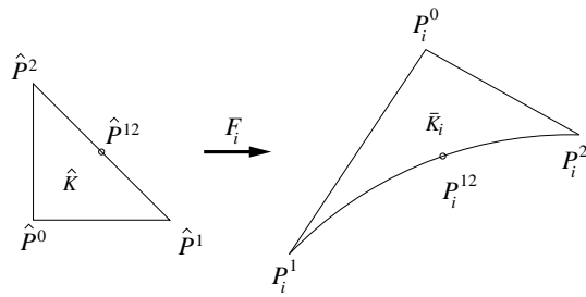
FIG. 5.7. Bilinear mapping F_i : \hat{K} \rightarrow K_i
